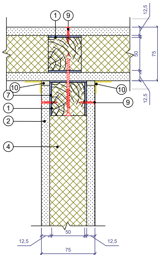
Примыкание перегородок под углом 90°
