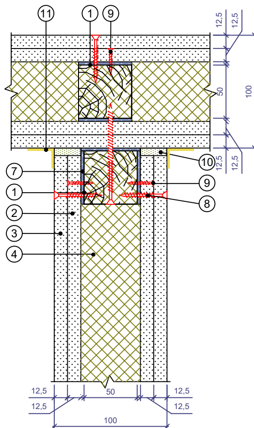
Примыкание перегородок под углом 90°
