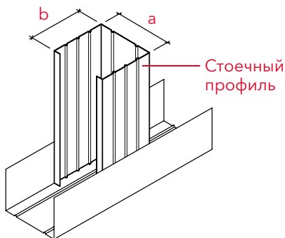
Геометрические размеры стойечных профилей
