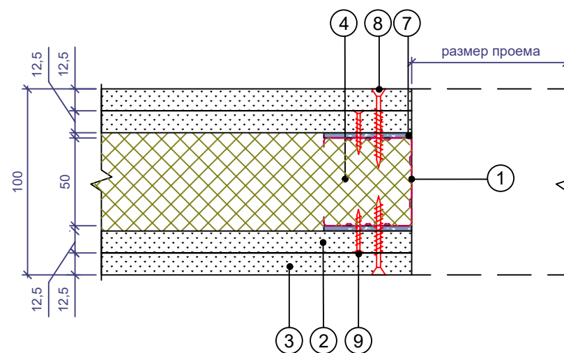
Стык перегородок
